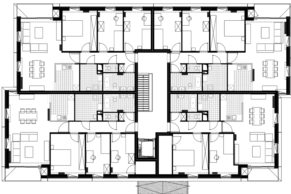
1e Verdieping appartementgebouw
